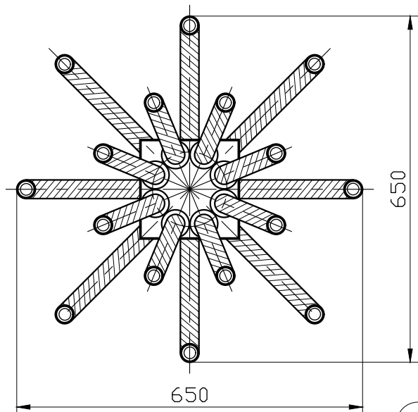
灯具平面図
