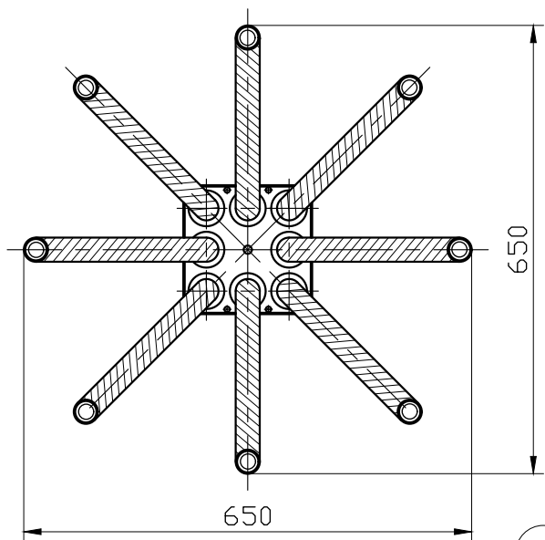
灯具平面图
