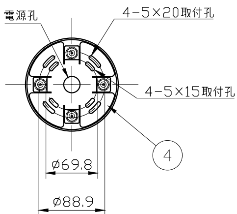
スタッド詳細 S=1/5
